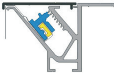
Spannrahmen "bleed" mit Abdeckung, Clip (blau) und Ausfüller (gelb)
