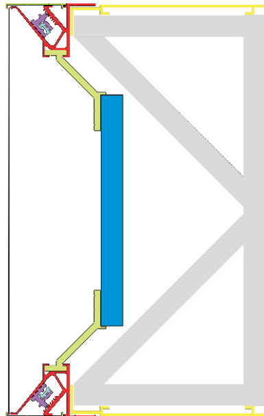
Spannrahmen bleed (rot); mit Stützprofil (grün) und Senkrechtstrebe 20 x 20 (blau). Beim Umrüsten einer vorhandenen Anlage entfällt die Notwendigkeit der grauen Stützkonstruktion.
